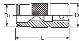
3131E Tap Holder Adaptadores para machos de terrajas
